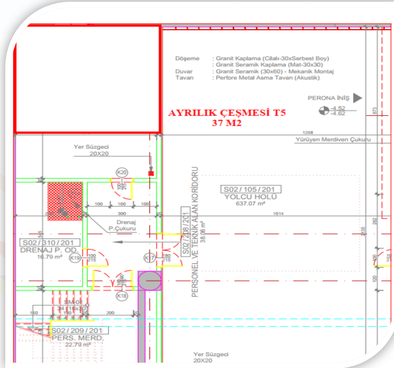
AYRILIK ÇEŞMESİ İSTASYONU BATI ARA KAT
