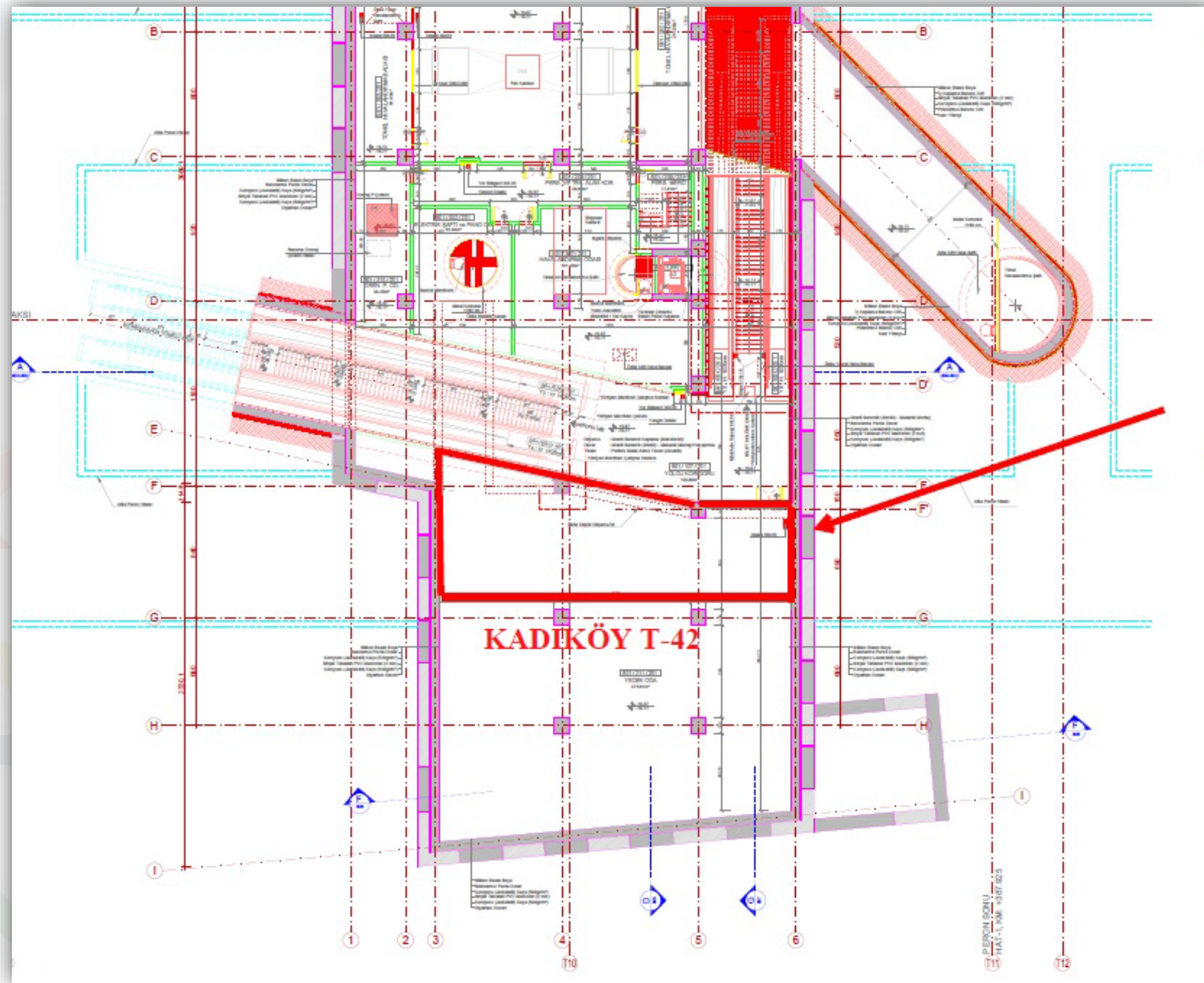
KADIKÖY İSTASYONU-DOĞU TURNİKE ARA KAT
