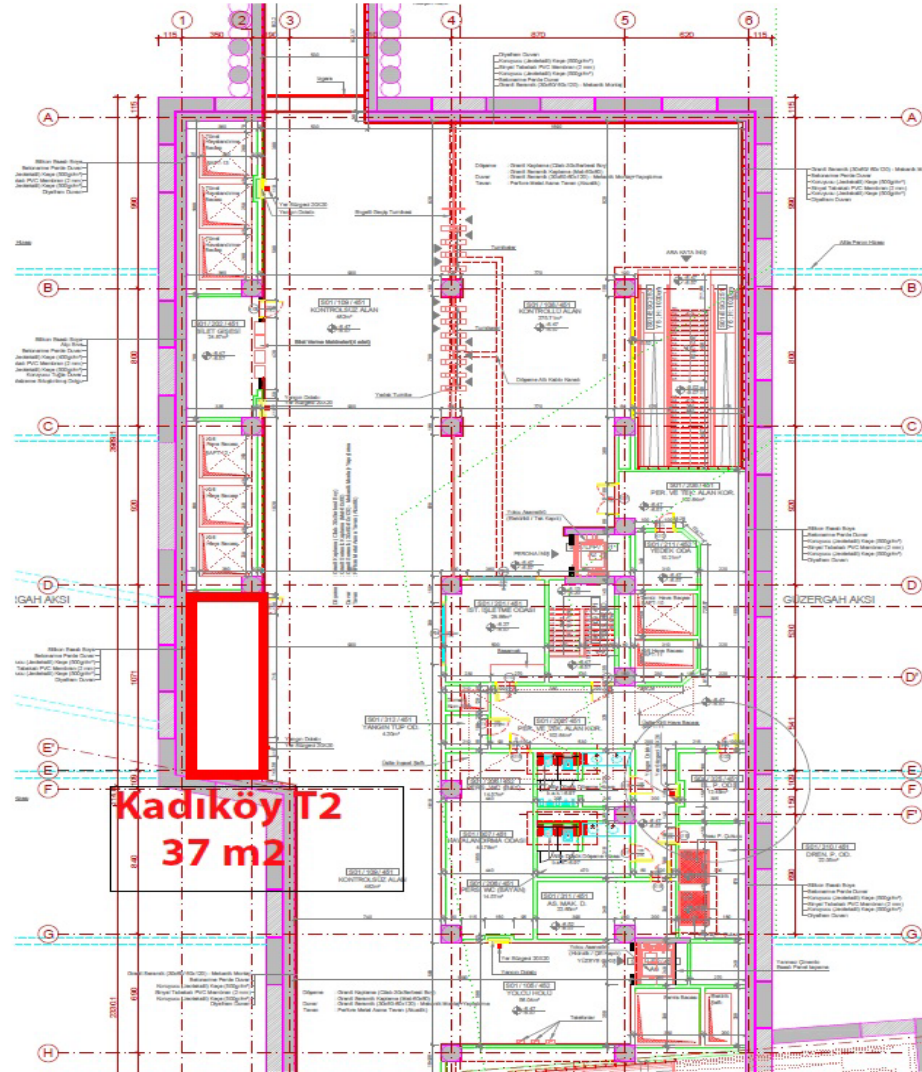
KADIKÖY İSTASYONU-DOĞU TURNİKE ARA KAT
